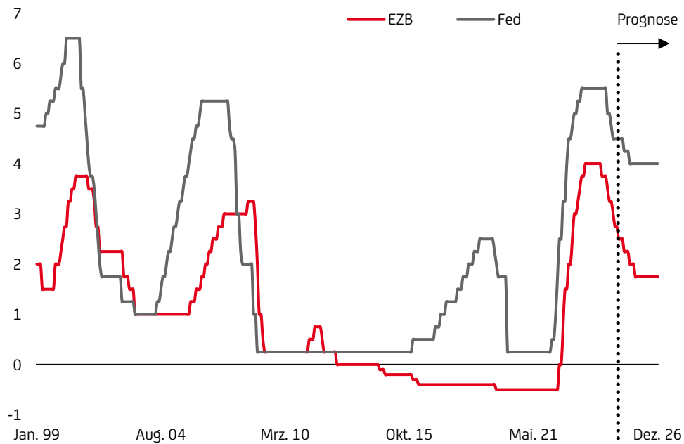
GRAFIK 1.2: TRANSATLANTISCHE ZINSDIFFERENZ DÜRFTE SICH AUSWEITEN LEITZINS, IN %
